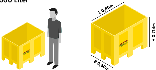
BATTERIESAMMELBOXEN 600 Liter
