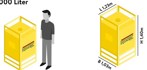
ASF BEHÄLTER 1000 Liter
