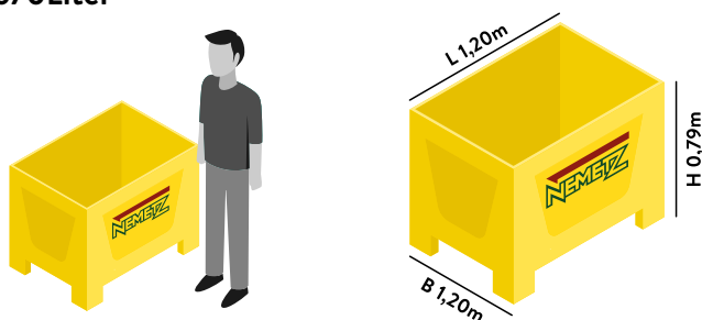
KUNSTSTOFFPALOXE 670Liter
