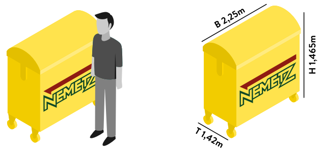
BEHÄLTER 2500 Liter
