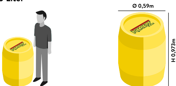
KUNSTSTOFFFASS 200 Liter
