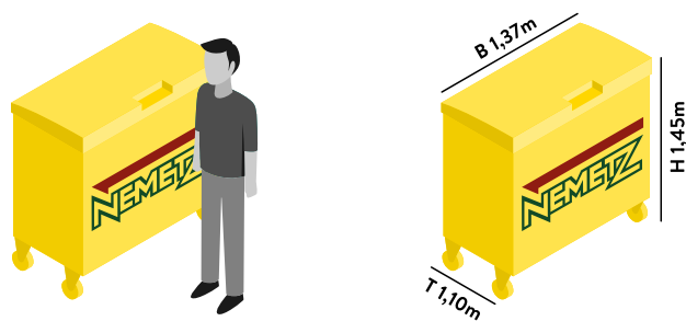
BEHÄLTER 1100 Liter
